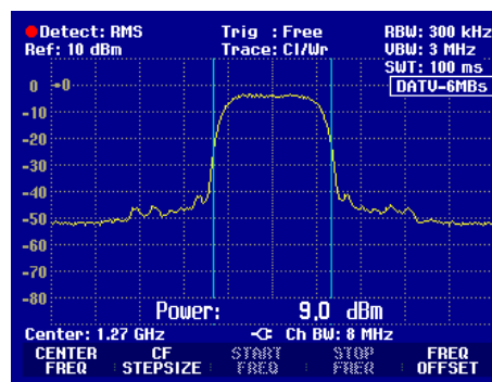
Spectre d'une émission DATV
