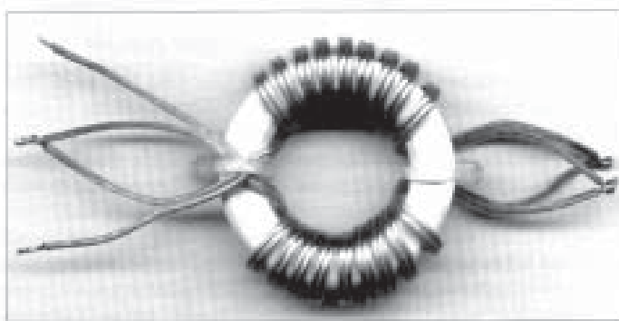
Bild 2: Nach DG0SA gewickelter 1:4-Balun, zur Messung vorbereitet
